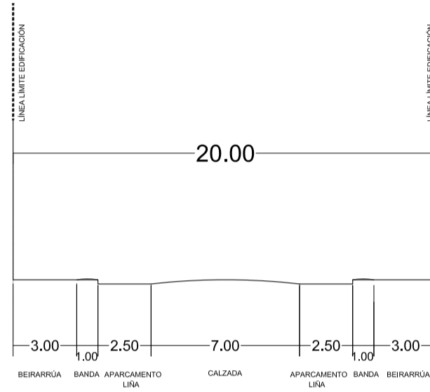
TIPO OU-5 ESTRADAS OU-0414 CP-0306
