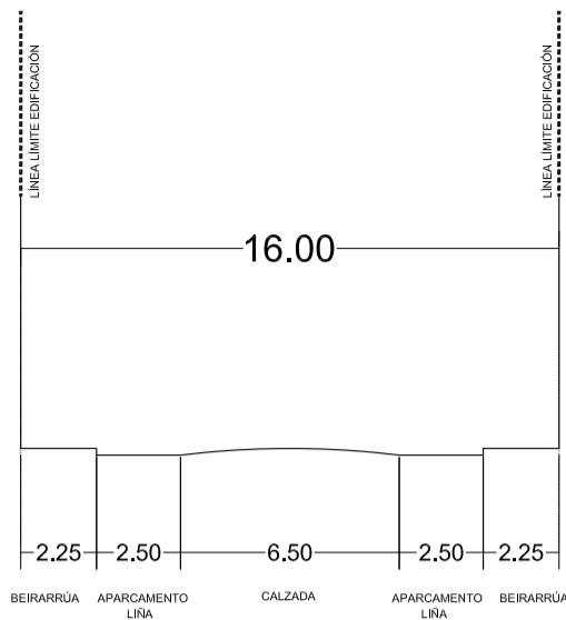
TIPO OU-4 ESTRADA OU-0307
