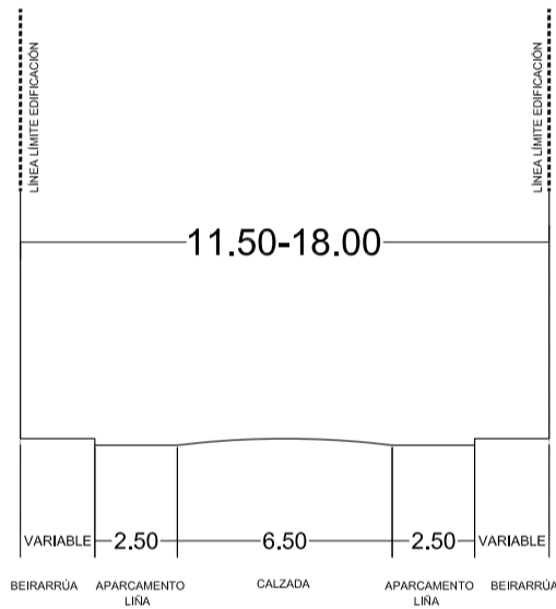
TIPO OU-6 ESTRADAS CP-4601 CP-4603
