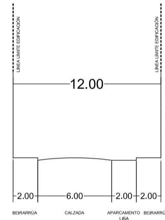
TIPO S.L.V.-2 DOUS SENTIDOS DE CIRCULACIÓN
