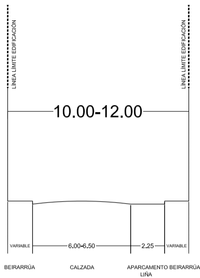
TIPO OU-1 ESTRADA OU-209
